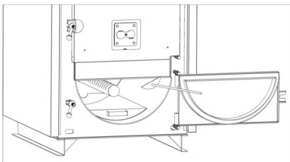
Fig 12. Καθαρισμός του εναλλάκτη
