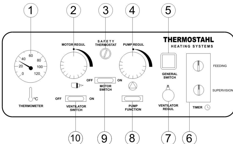
Fig 7. Πίνακας ελέγχου
