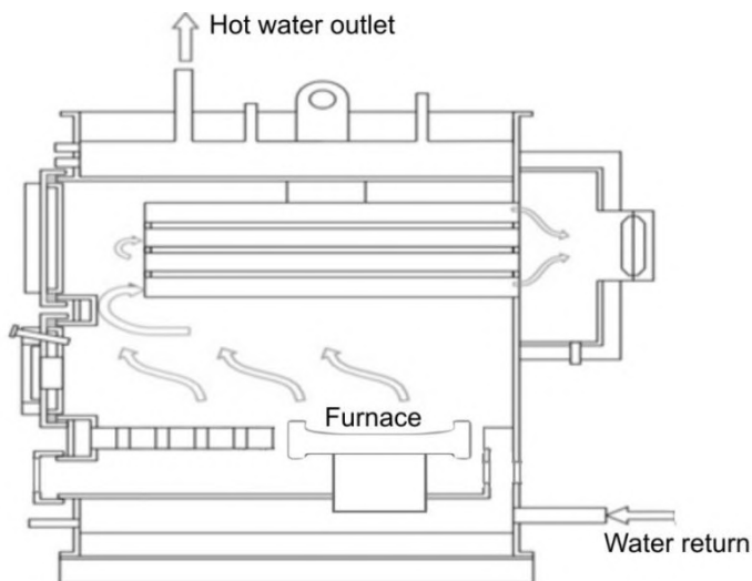
Fig 1. Λειτουργία λέβητα
