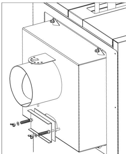
Fig 14. Καθαρισμός καπνοσυλλέκτη
