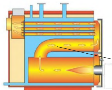
Βρεχόμενη 2η διαδρομή καυσαερίων
