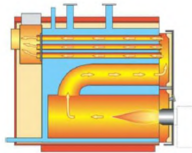
Σχεδιάγραμμα λειτουργίας λέβητα Pelletstar με τρεις διαδρομές καυσαερίων
